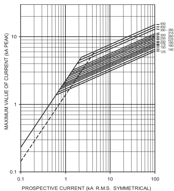
Caratteristiche di limitazione 3LS - Cut-off characteristics 3LS
